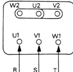
Conexión Estrella
