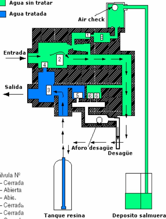
C0 Posición agua tratada Posición de servicio
